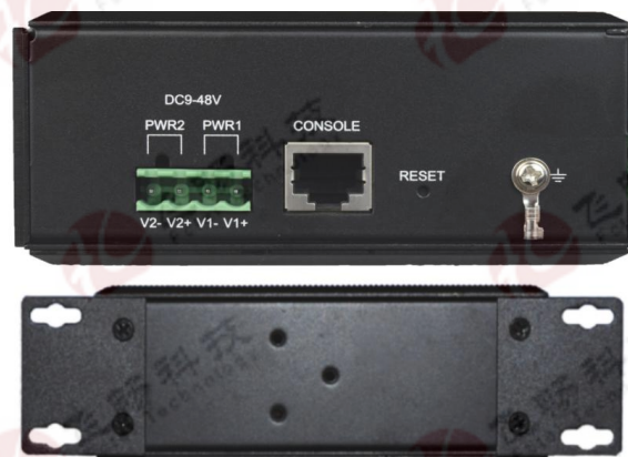
壁挂式安装
